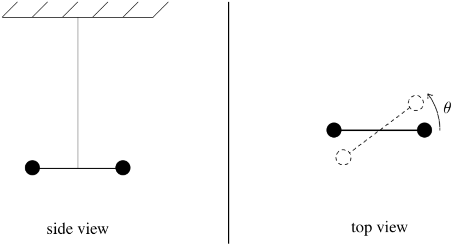
Figura 1.14: dos vistas de un péndulo de torsión —una barra o mancuerna suspendida por su centro mediante un hilo o fibra desde un soporte superior; la vista superior muestra el ángulo de torsión \theta .
