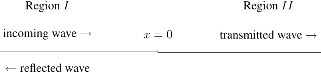
Figura 9.1: dos cuerdas semiinfinitas unidas en x = 0 ; en la región I, a la izquierda, hay una onda entrante hacia la derecha y una reflejada hacia la izquierda; en la región II, a la derecha, hay una onda transmitida hacia la derecha.
