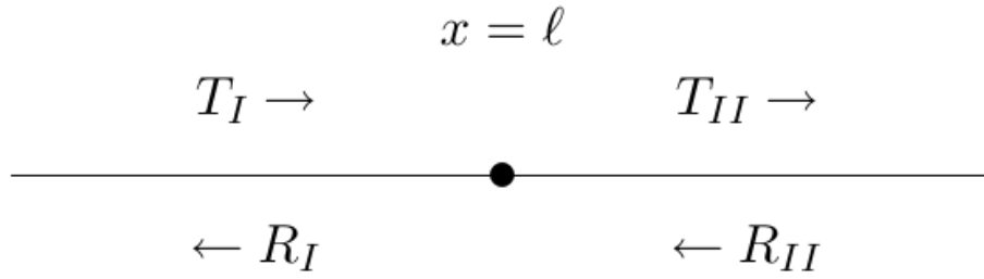
Figura 9.6: el problema general de dispersión debido a una única masa en x = \ell , con ondas entrante y saliente a ambos lados, T_I, R_I a la izquierda y T_{II}, R_{II} a la derecha.
