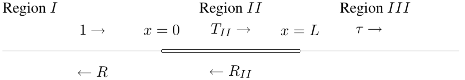
Figura 9.9: reflexión en una película delgada, con tres regiones: I ( x \leq 0 , con onda entrante 1 y reflejada R), II ( 0 \leq x \leq L , con T_{II} , R_{II} ) y III ( x \geq L , con onda transmitida \tau ).
