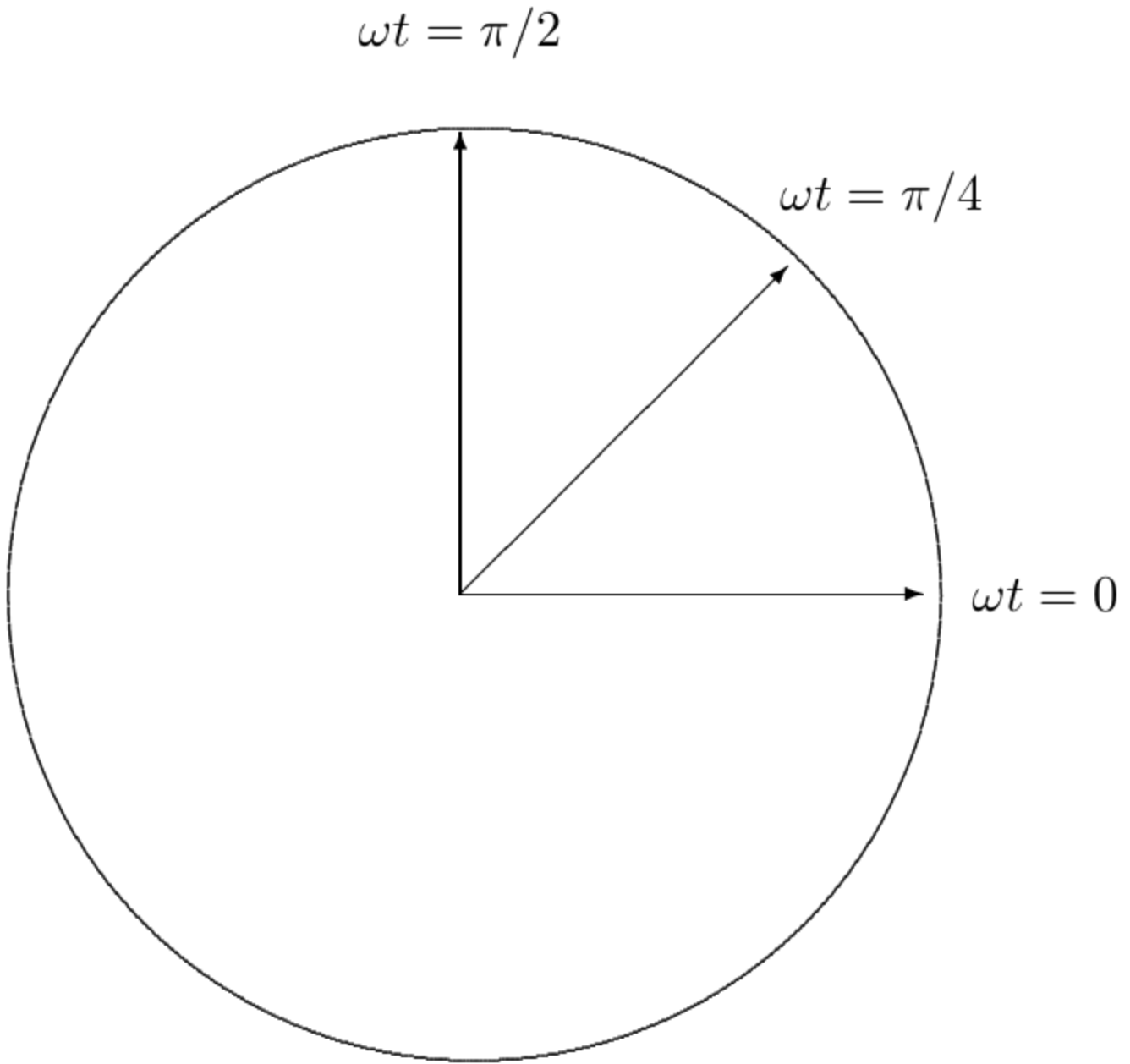
Figura 12.2: polarización circular.
