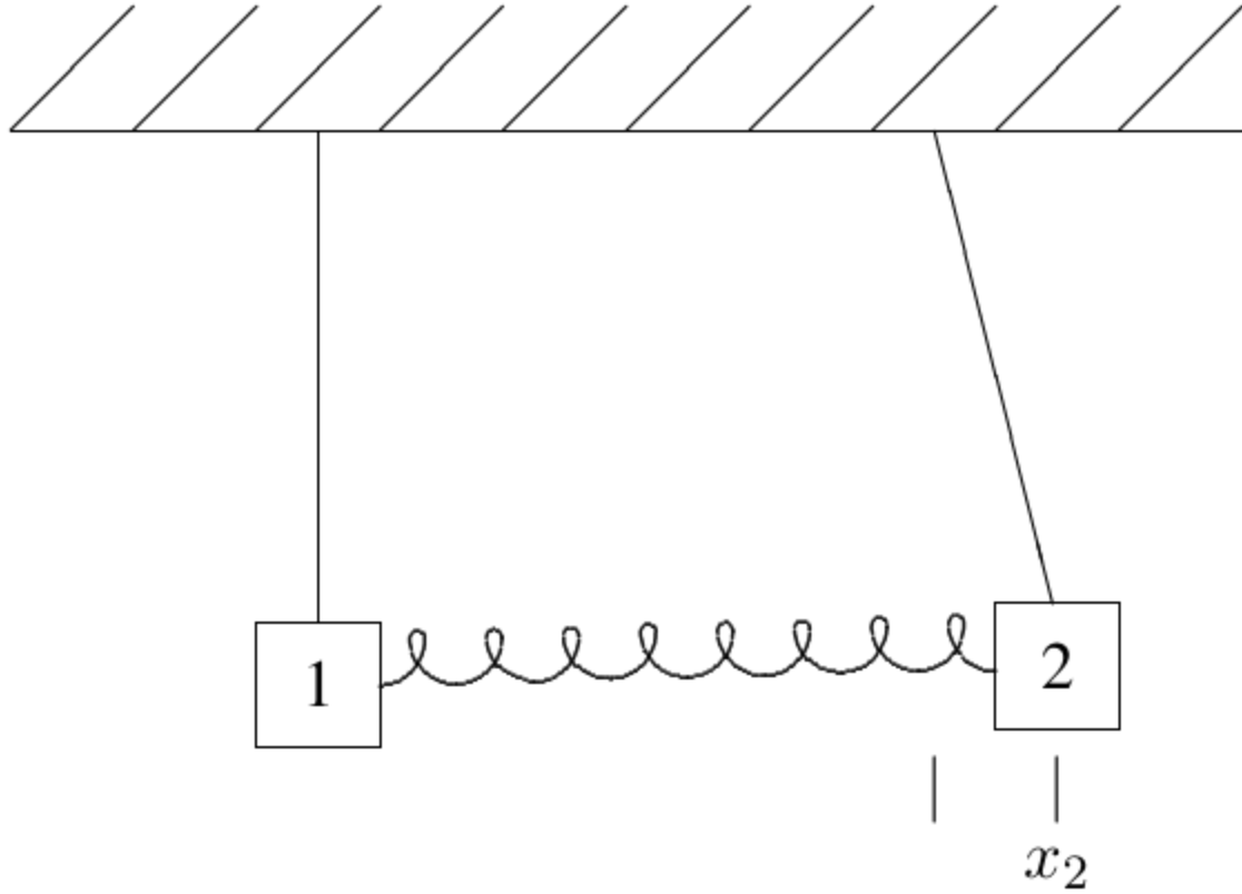
Figura 3.3: los dos péndulos con el bloque 2 desplazado una cantidad x_2 y el bloque 1 mantenido en su posición de equilibrio.
