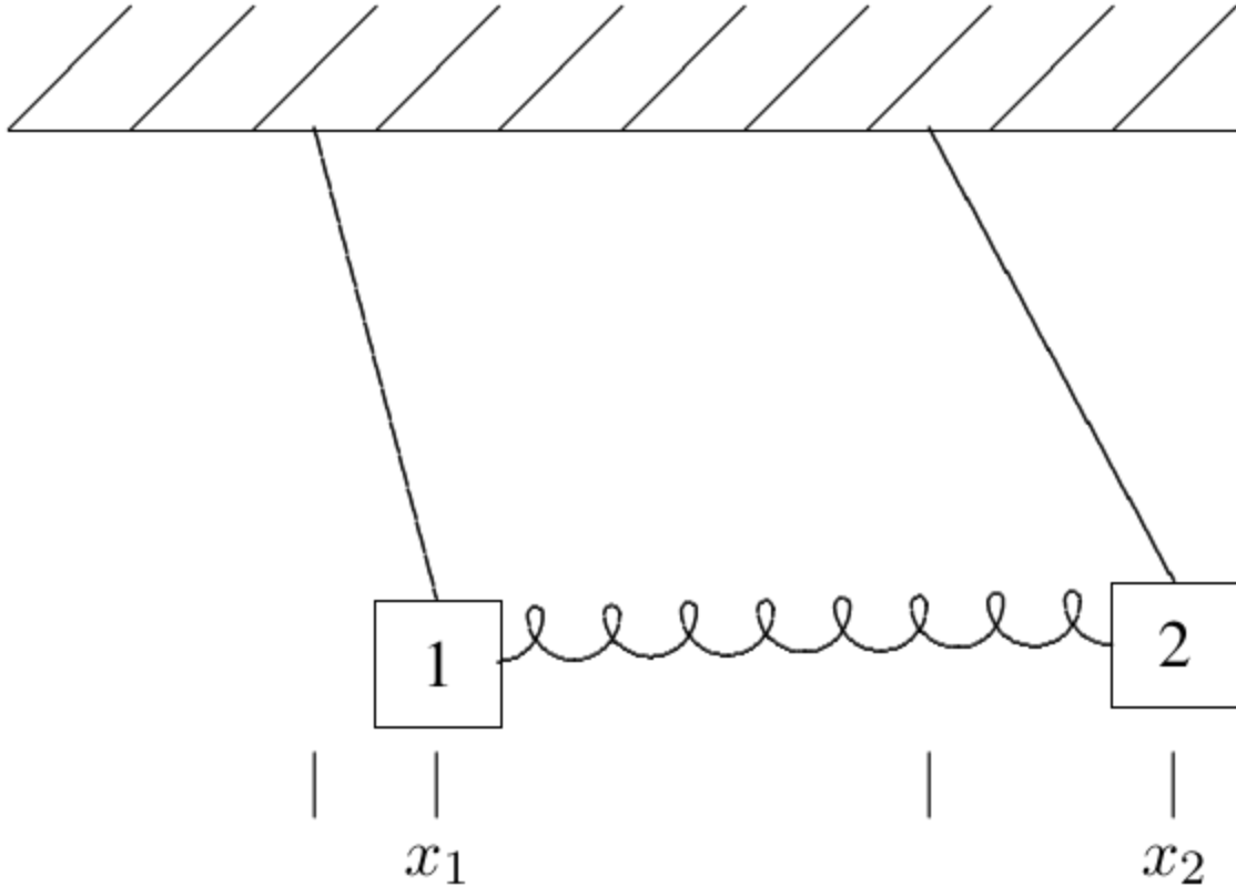
Figura 3.2: los mismos dos péndulos, ahora desplazados de su posición de equilibrio en las cantidades horizontales x_1 y x_2 .
