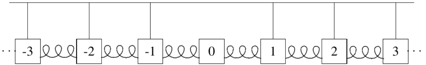
Figura: cadena infinita de péndulos acoplados numerados \dots, -3, -2, -1, 0, 1, 2, 3, \dots ; el péndulo 0 puede deslizarse longitudinalmente sin fuerza restauradora gravitatoria, solo con el acoplamiento de los muelles.
