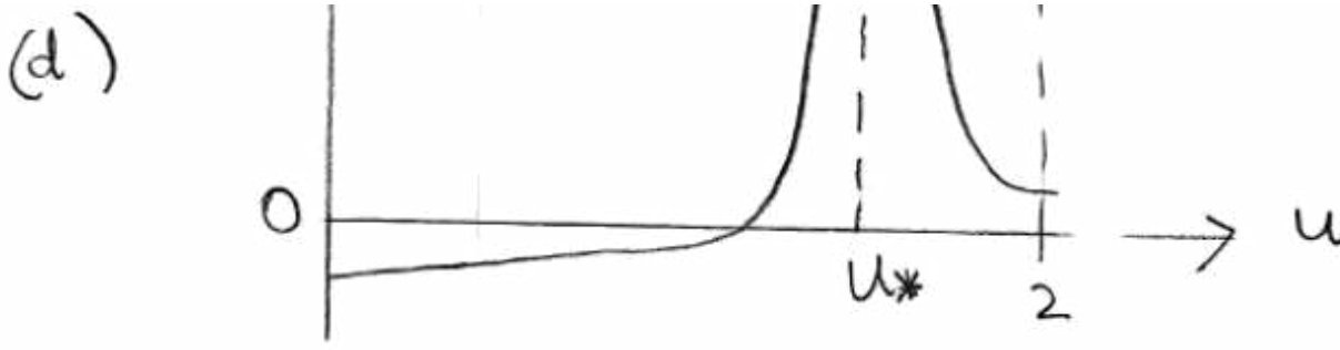
Figura 5: Gráfico de varias cantidades en función de u = ka , con el potencial caracterizado por z_0^2 = 1 y z_1^2 = 5 . (a) \delta(E) aumenta rápidamente alrededor de u_* = 1.85 , o equivalentemente E = 0.69 V_1 , cruzando -\pi/2 y señalando comportamiento resonante. (b) Gráfico de |A_s|^2 = \sin^2 \delta , mostrando picos cada vez que |\delta| = \pi/2 . (c) El coeficiente |A| de la función de onda en el pozo alcanza su pico en la resonancia, mostrando alta probabilidad de encontrar la partícula en el pozo. (d) El retraso temporal es positivo y alcanza su pico en la resonancia.
