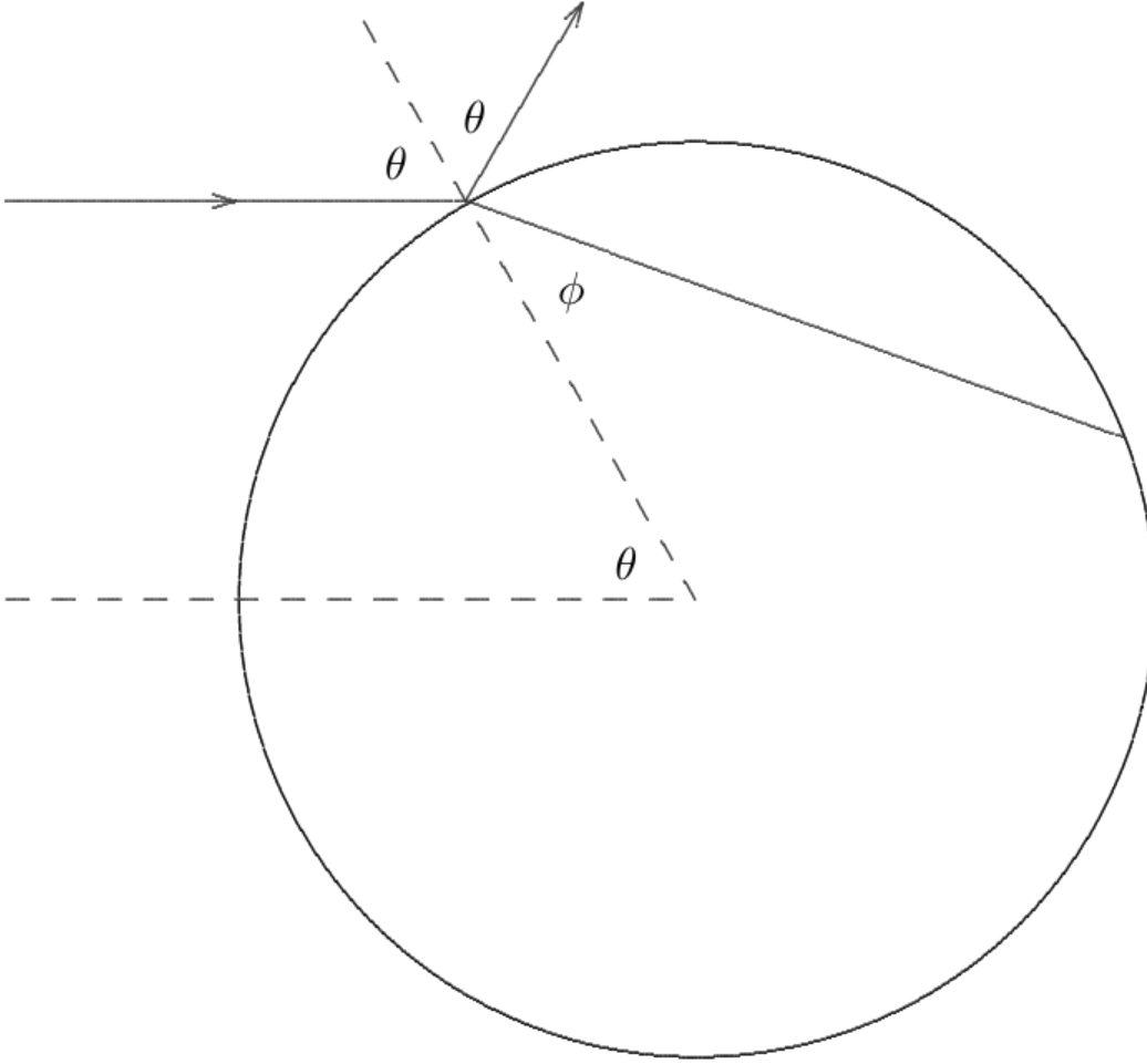
Figura 11.50: refracción de un rayo en una gota esférica.
