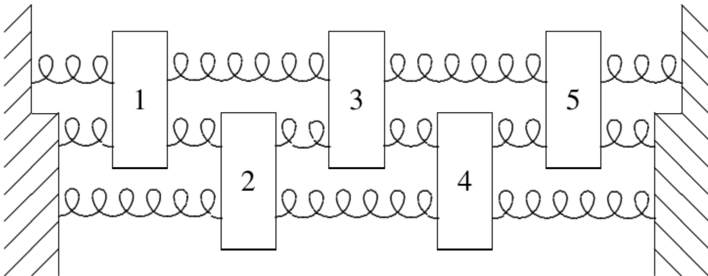
Figura: cinco bloques en línea entre dos paredes fijas, conectados por una alternancia de muelles largos (constante K ), medianos (constante 2K ) y cortos (constante 3K ), en un patrón simétrico.
