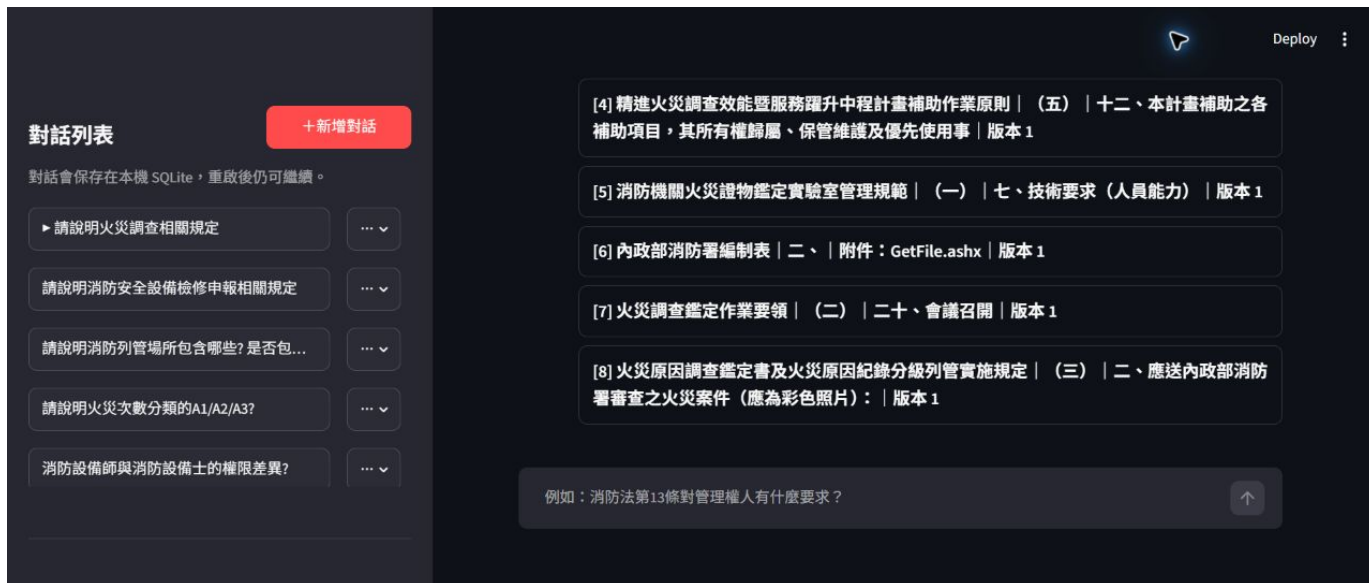
圖 3 成功回答中的引用編號與展開的法規證據卡
