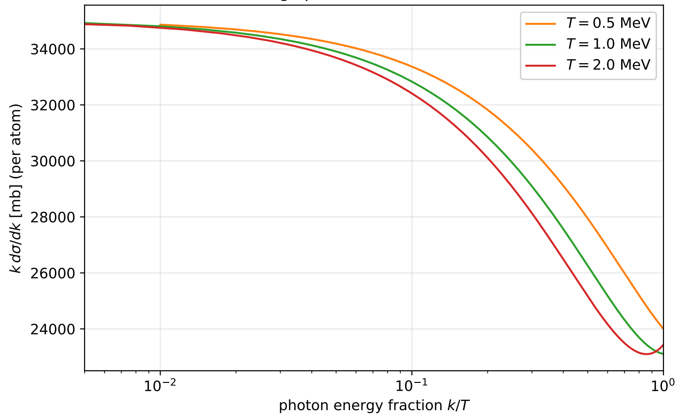
Bremsstrahlung spectrum in Xe (Bethe-Heitler-Tsai)
