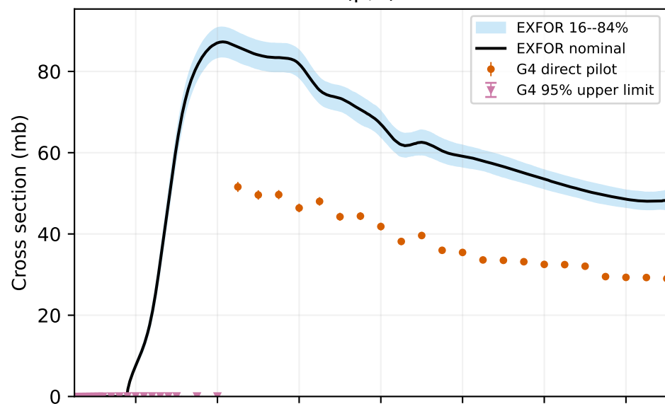
C-12(p,x)C-11
