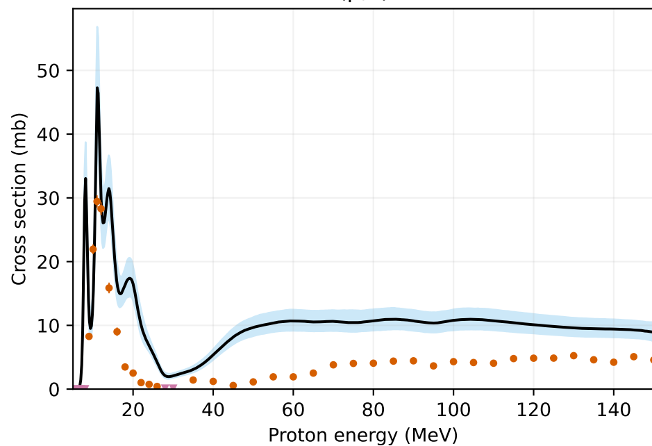
O-16(p,x)N-13
