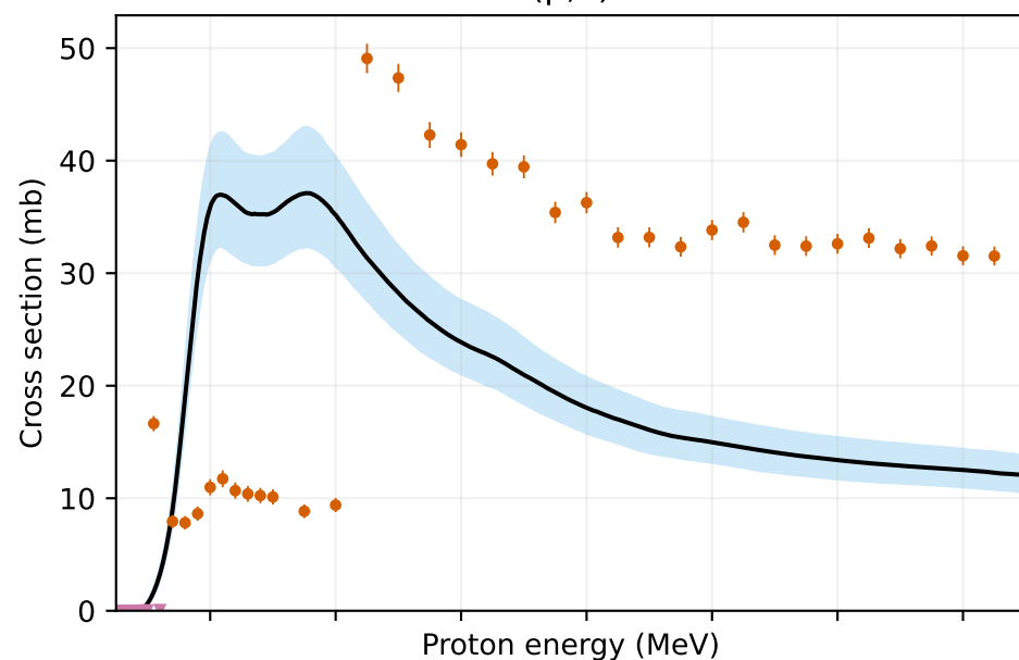
N-14(p,x)N-13
