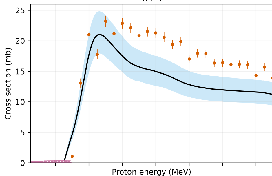
O-16(p,x)N-13
