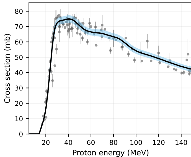
O-16(p,x)N-13
