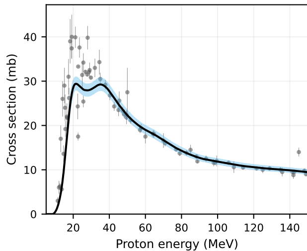
N-14(p,x)N-13
