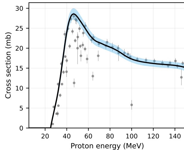
O-16(p,x)C-11
