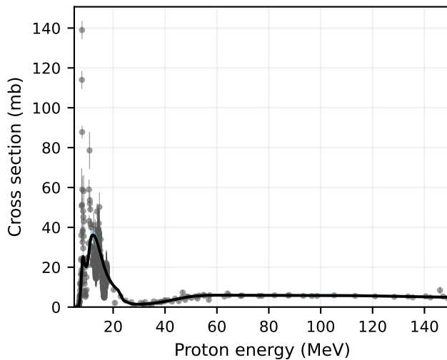
O-16(p,x)N-13
