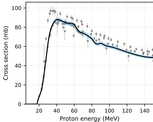
N-14(p,x)N-13
