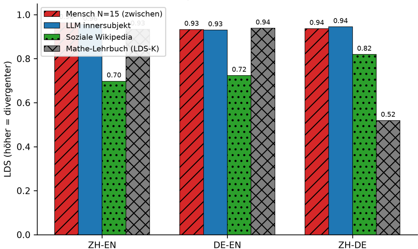
Abb. 12 — Drei-Ebenen-Vergleich (Rohwerte). Mensch (N=15, between) vs. LLM (within) vs. soziale Wikipedia vs. Lehrbuch — gleiche Signalamplitude Mensch/LLM (0,93 – 0,96), unterschiedliche Böden. Lehrbuch-ZH-DE T1-falsifiziert.
