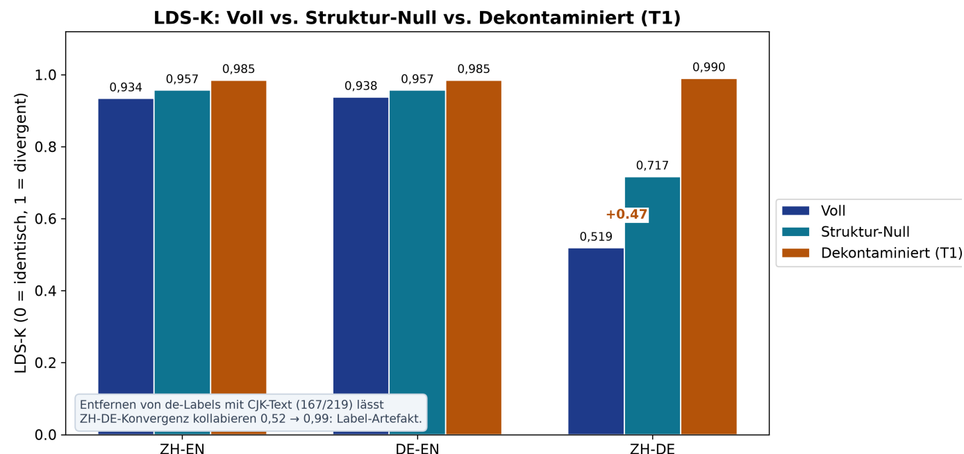
Abb. 10 — Dekontamination (T1 FilterA). Entfernen CJK-kontaminierter de-Labels (167/219, 52 behalten): ZH-DE 0,52→0,99 (J 0,556→0,020, Pfeil +0,47). Deterministischer Snapshot ohne Recompute.
