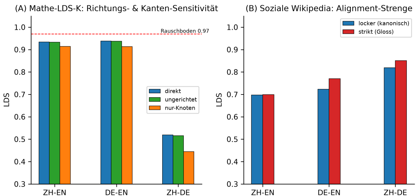
Abb. 8 — Sensitivität. (A) Richtungs-/Kanten-Robustheit mit Rauschboden 0,97; (B) Wiki-Alignmentstrenge (locker vs. strikt). Rangfolge stabil.
