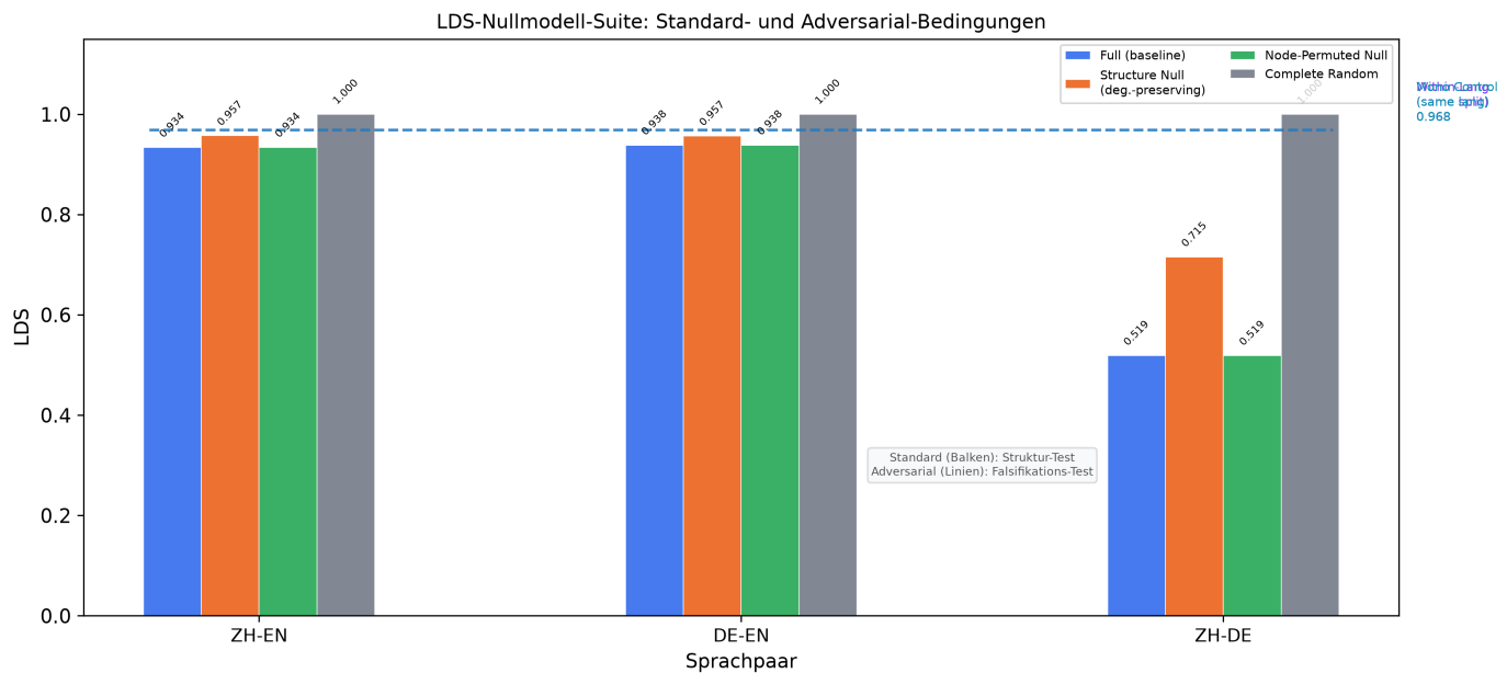
Abb. 7 — LDS-K gegen Nullmodelle. Full < Struktur-Null für alle Paare (deskriptiv); ZH-DE 0,519 T1-falsifiziert (dekontaminiert 0,99). Snapshot 2026-09-12 + Re-Freeze 2026-09-16 ( \delta im Rundungsband); Struktur-Null-Punkt 0,715 (5-seed-Mittel 0,717).
