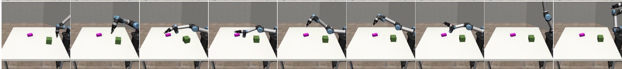
PPO+RND
