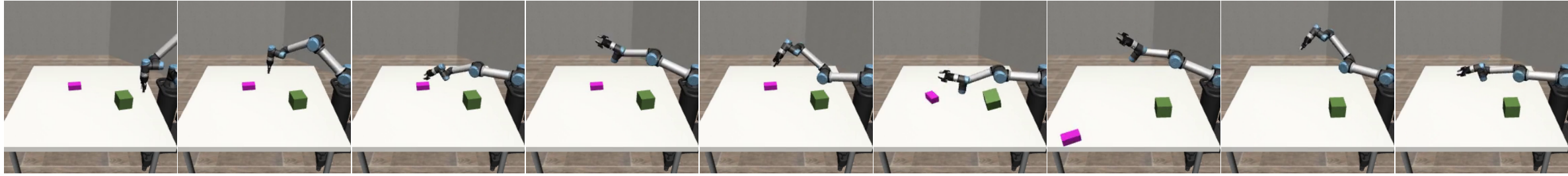
DreamerV3
