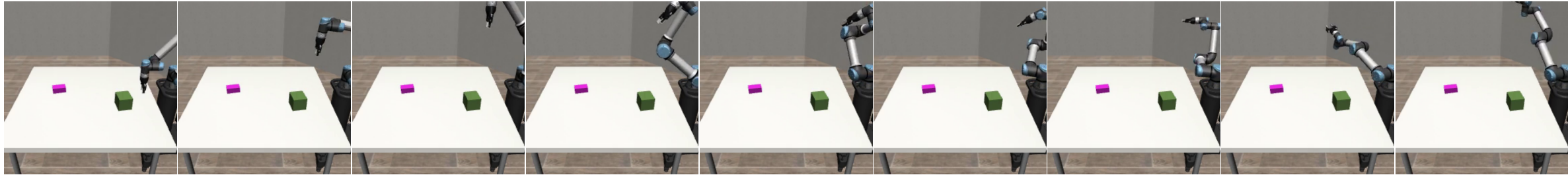
SAC
