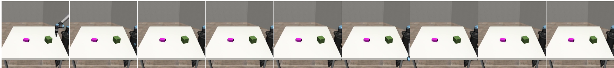
PPO
