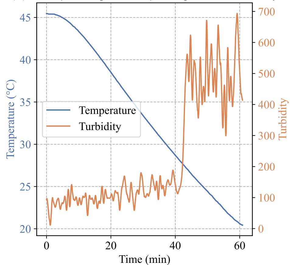
(D) 0.3 \text{ }^\circ\text{C}/\text{min} - Temperature & Turbidity
