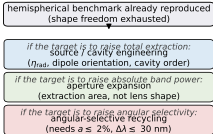
(d) design-route map
