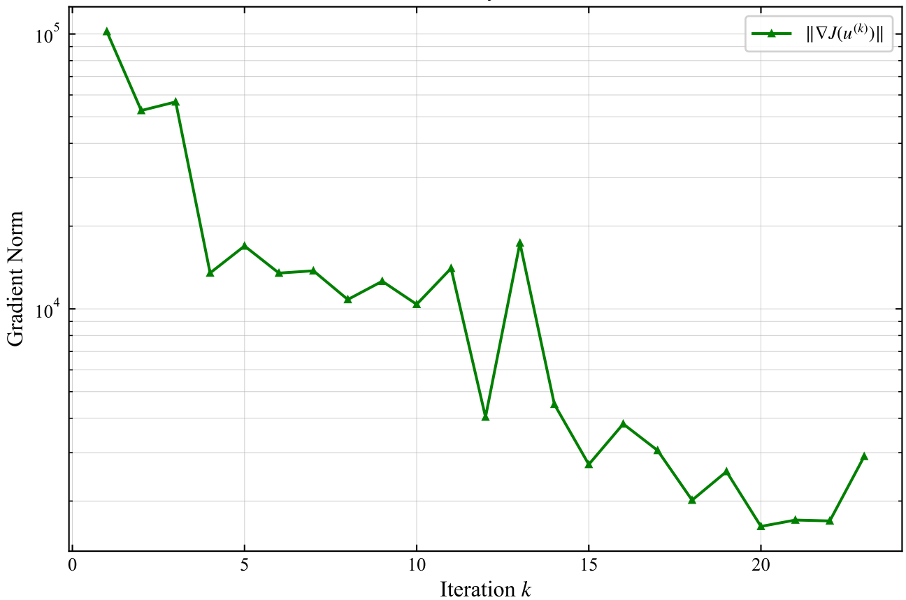
Gradient Norm History — GradientDescent
