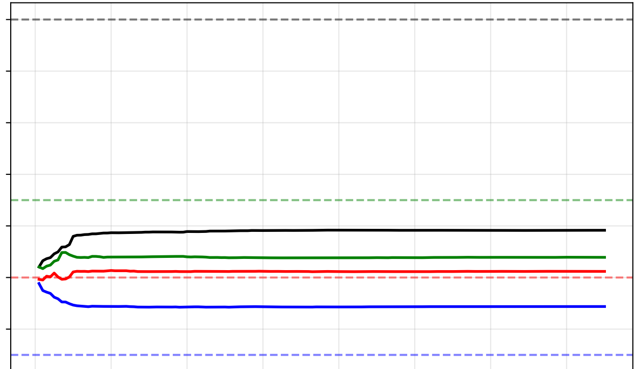
Planet B
