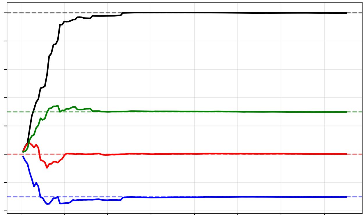
Planet D
