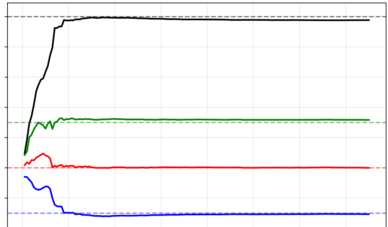
Planet B
