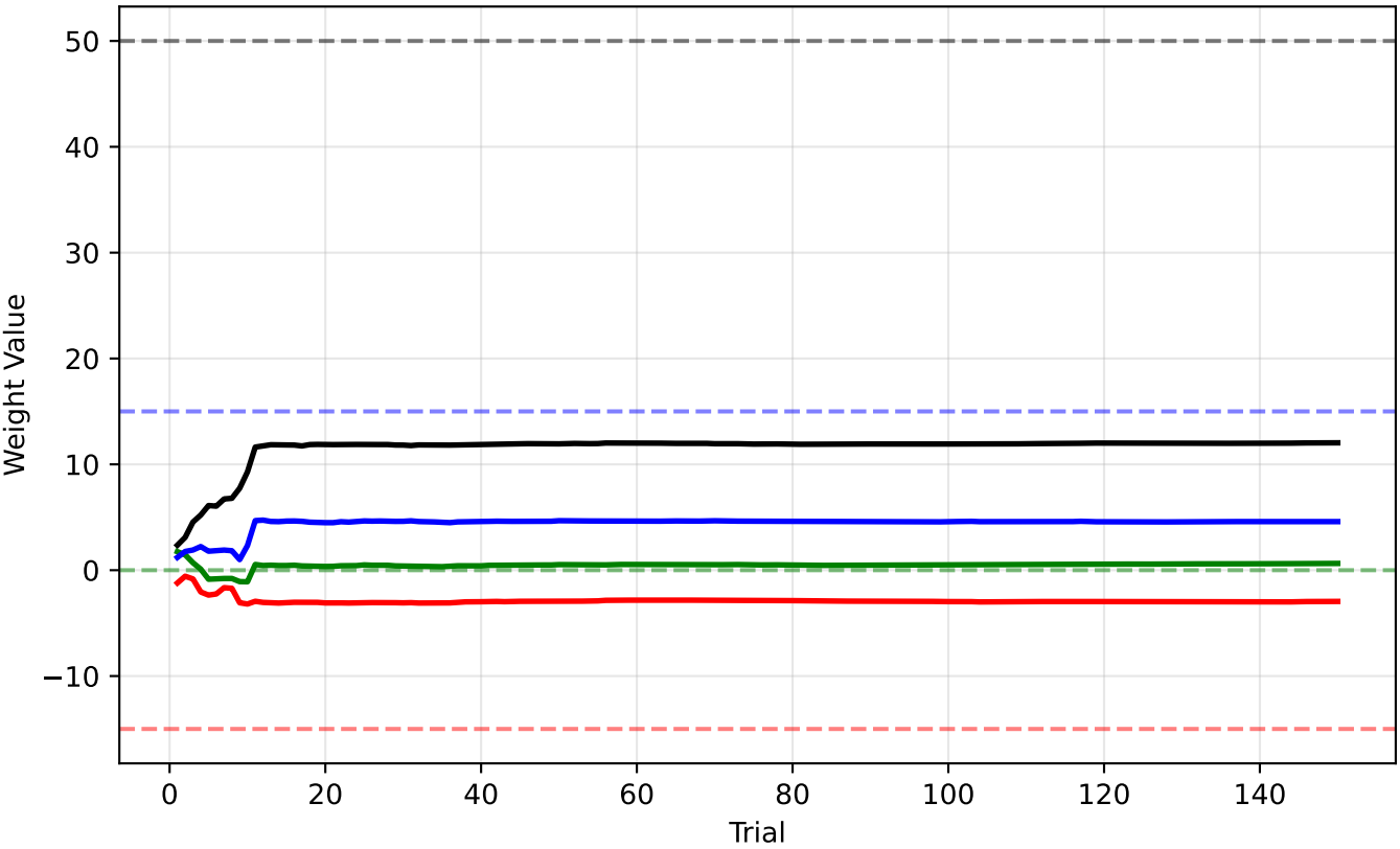
Planet C
