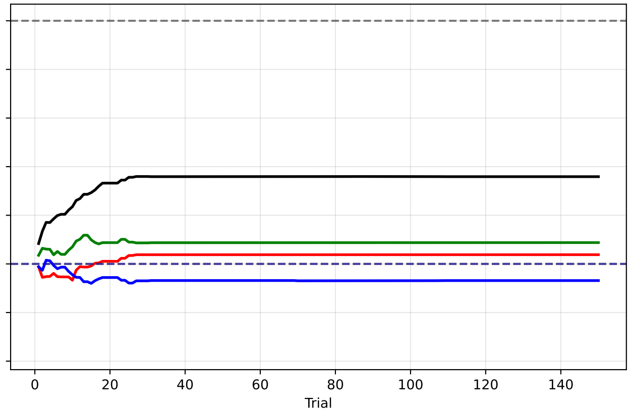
Planet D
