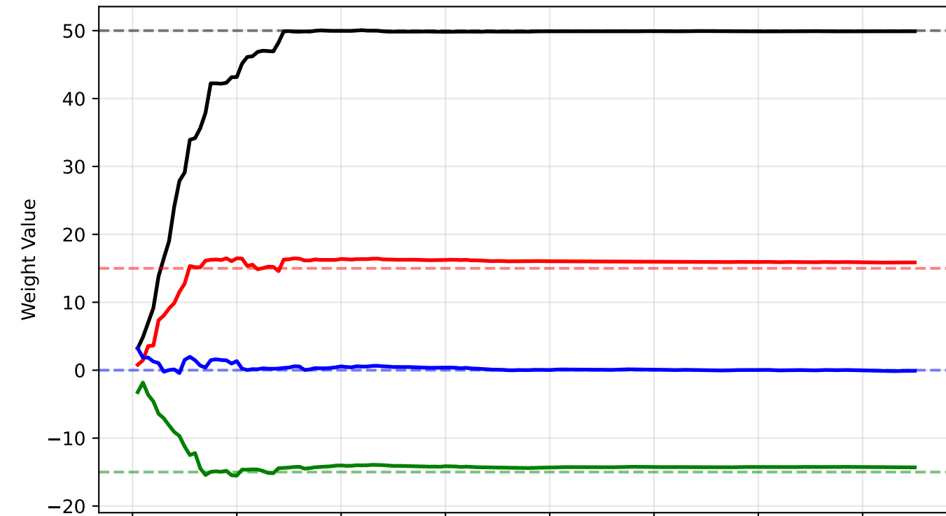
Planet C
