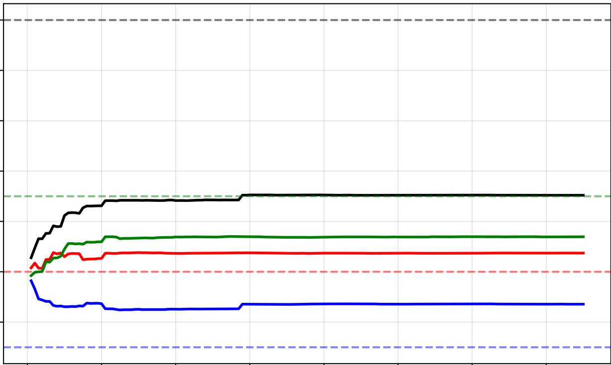
Planet B
