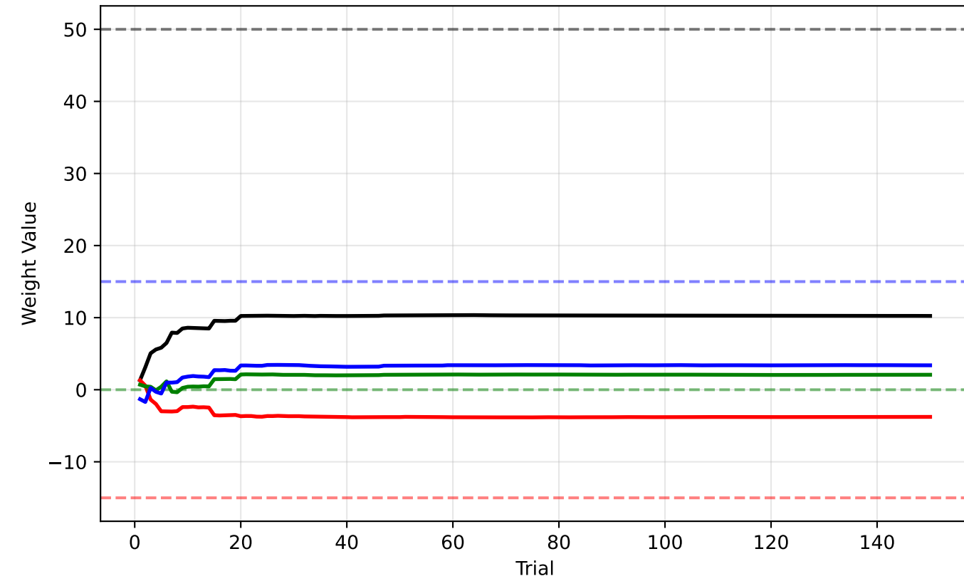
Planet C
