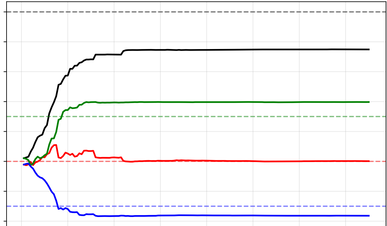
Planet B
