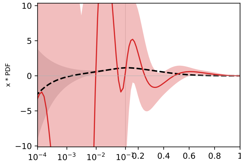
g (gluon)
