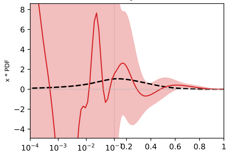
g (gluon)
