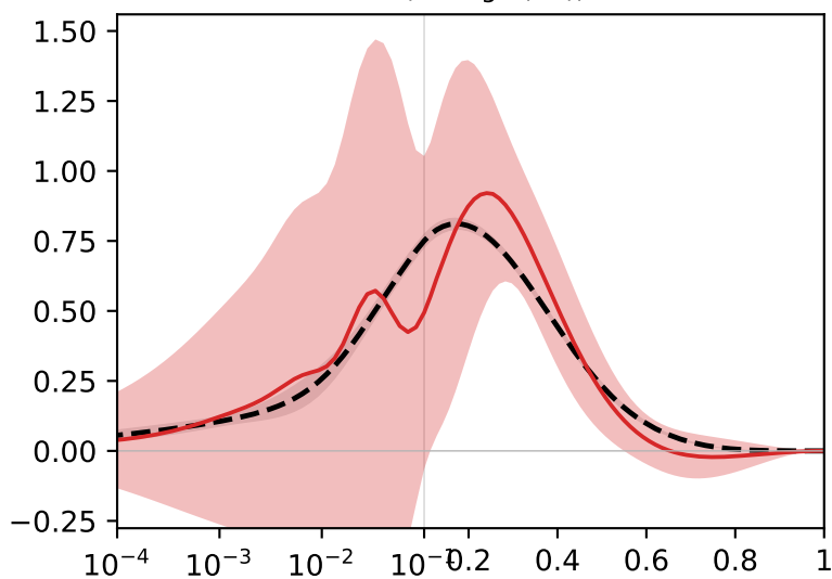
v8 (strange (V8))
