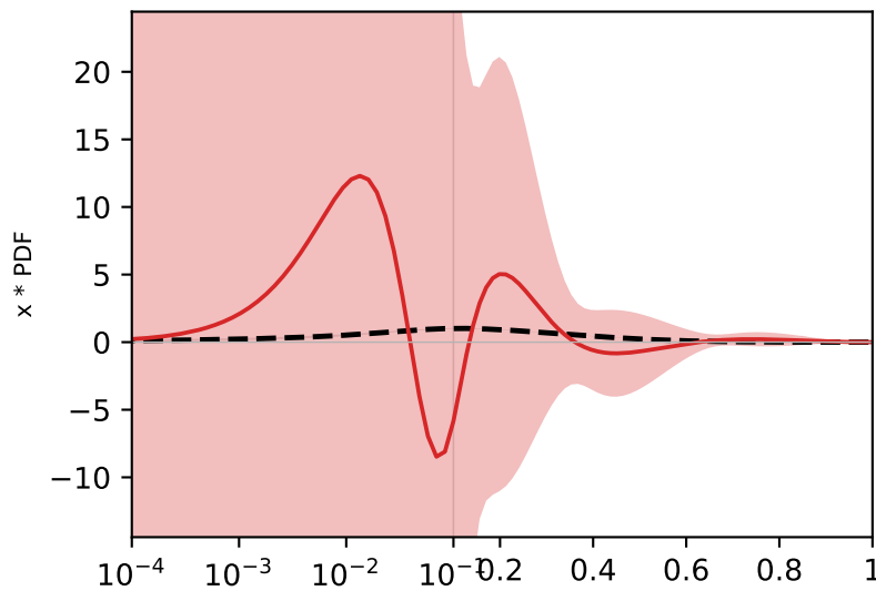
g (gluon)
