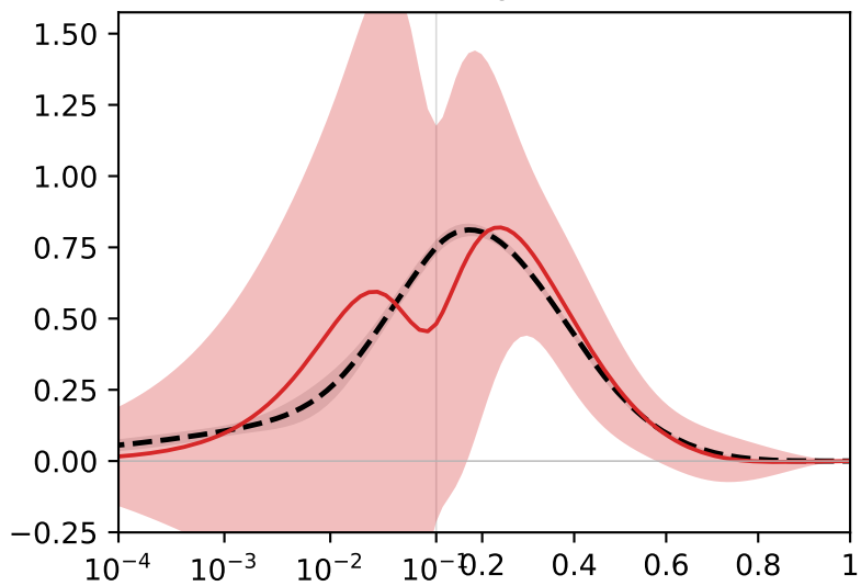
v8 (strange (V8))
