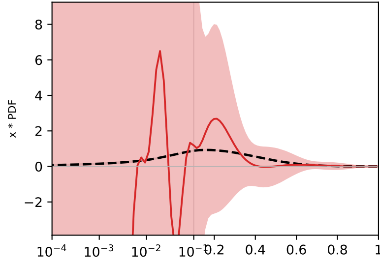
g (gluon)
