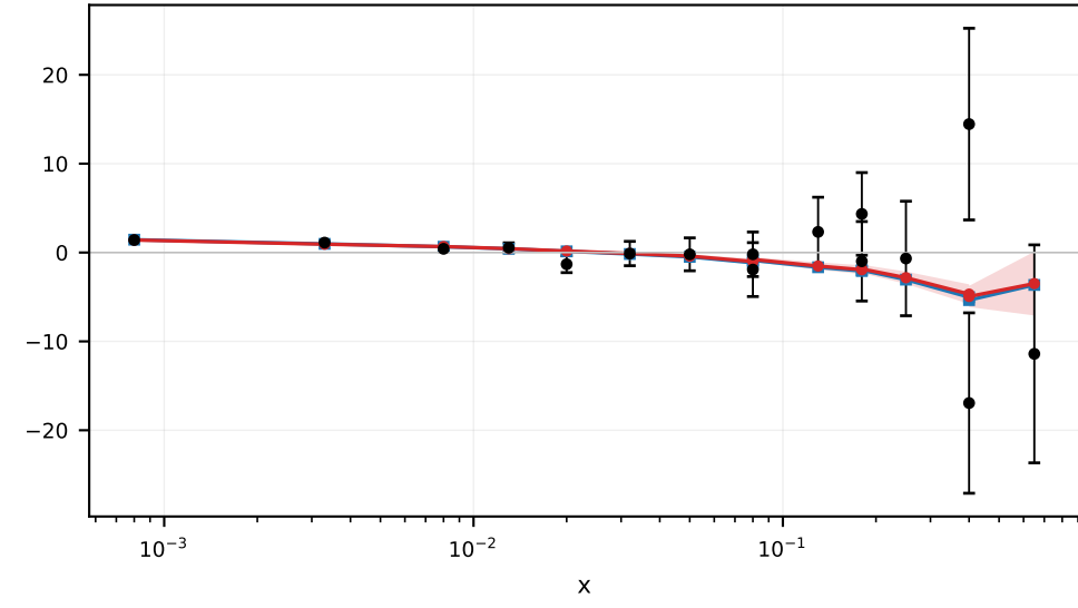
slac_p_f2 chi2/n=0.62 n=16
