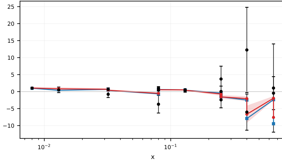
hera_nc_ep_318_sigmar chi2/n=0.46 n=16
