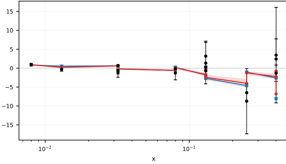
slac_d_f2 chi2/n=0.52 n=16
