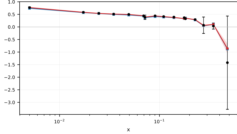
nmc_p_f2 chi2/n=0.38 n=16
