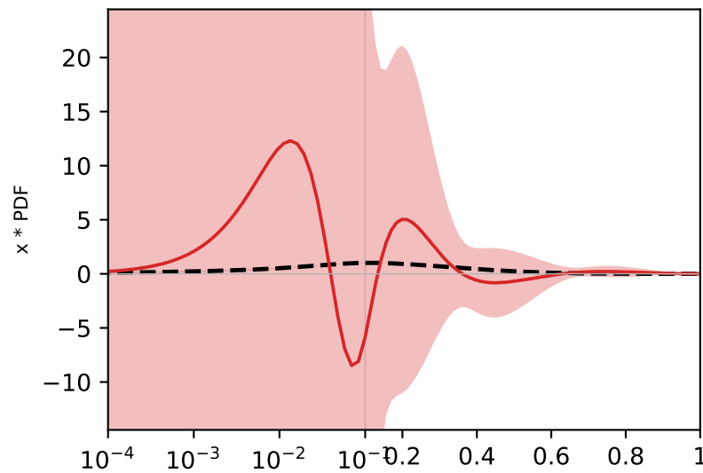
g (gluon)
