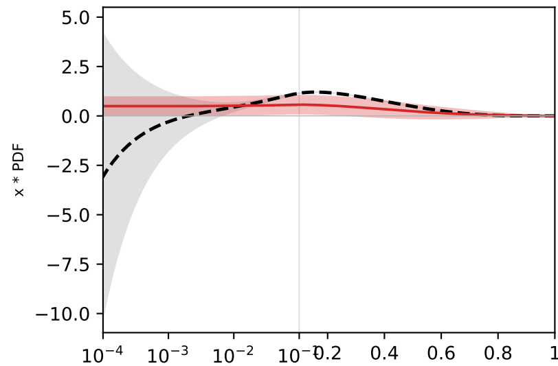
g (gluon)
