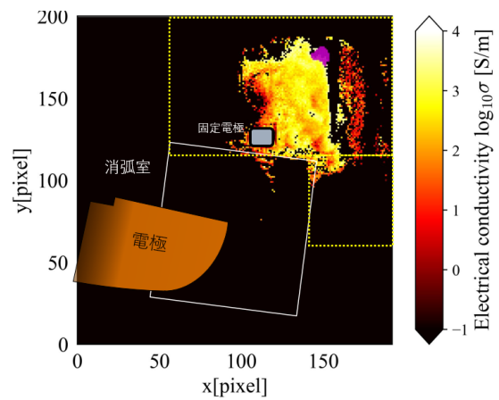
(d2) ケース b の導電率
