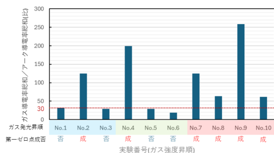
ガス導電率総和／アーク導電率総和(比)
