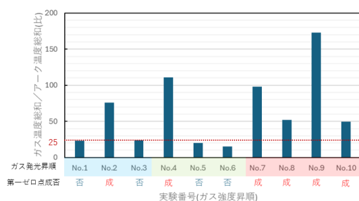
ガス温度総和／アーク温度総和(比)
