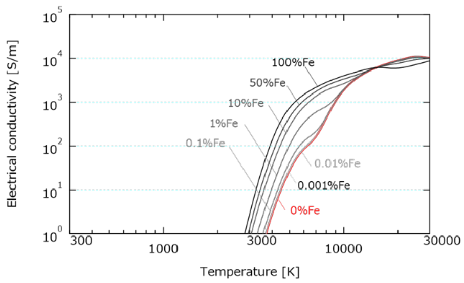
図 3.2.7 鉄蒸気混入空気の導電率 \sigma ( p = 1 \text{ bar} )
