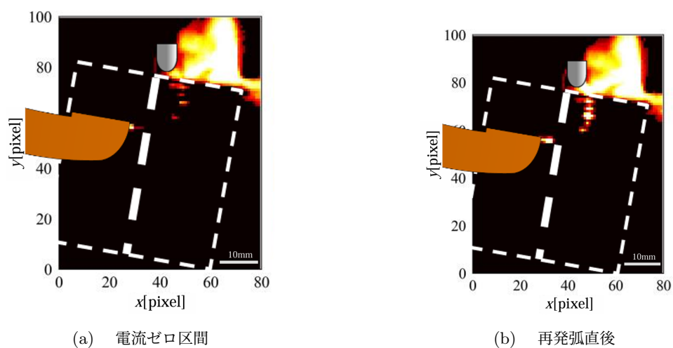
図 1.1.1 熱的再発弧時の発光画像
