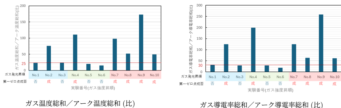
図 4.2.11 各実験番号におけるガス - アーク温度・導電率総和比
