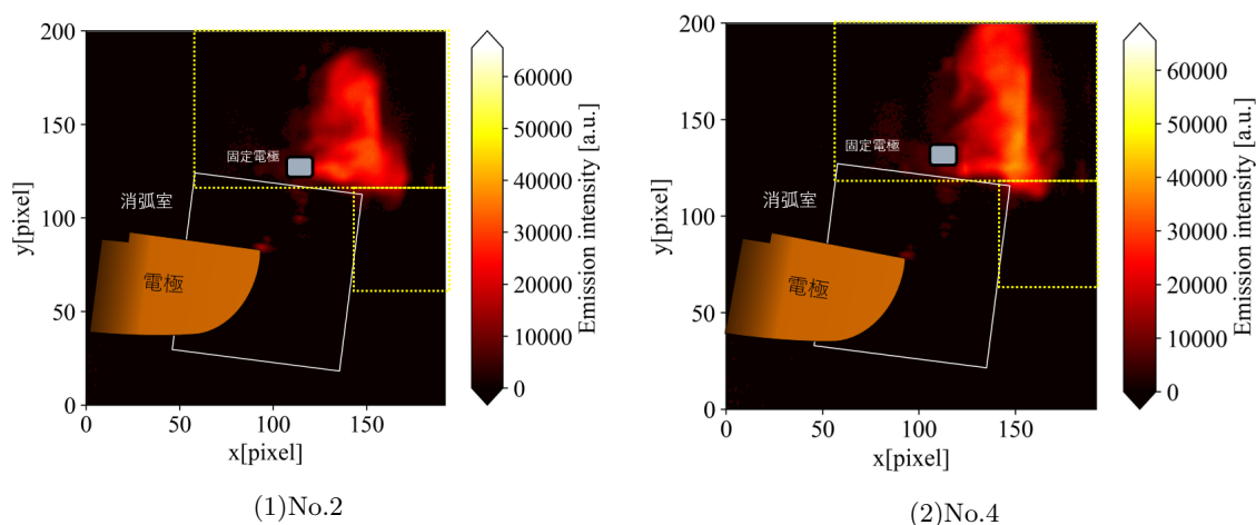
図 4.2.12 No.2, No.4 の発光画像
