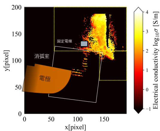
(c2) ケース a の導電率
