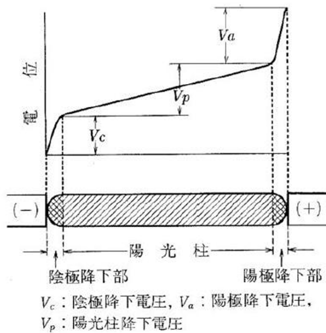
図 2.1.1 アーク放電の電位分布
