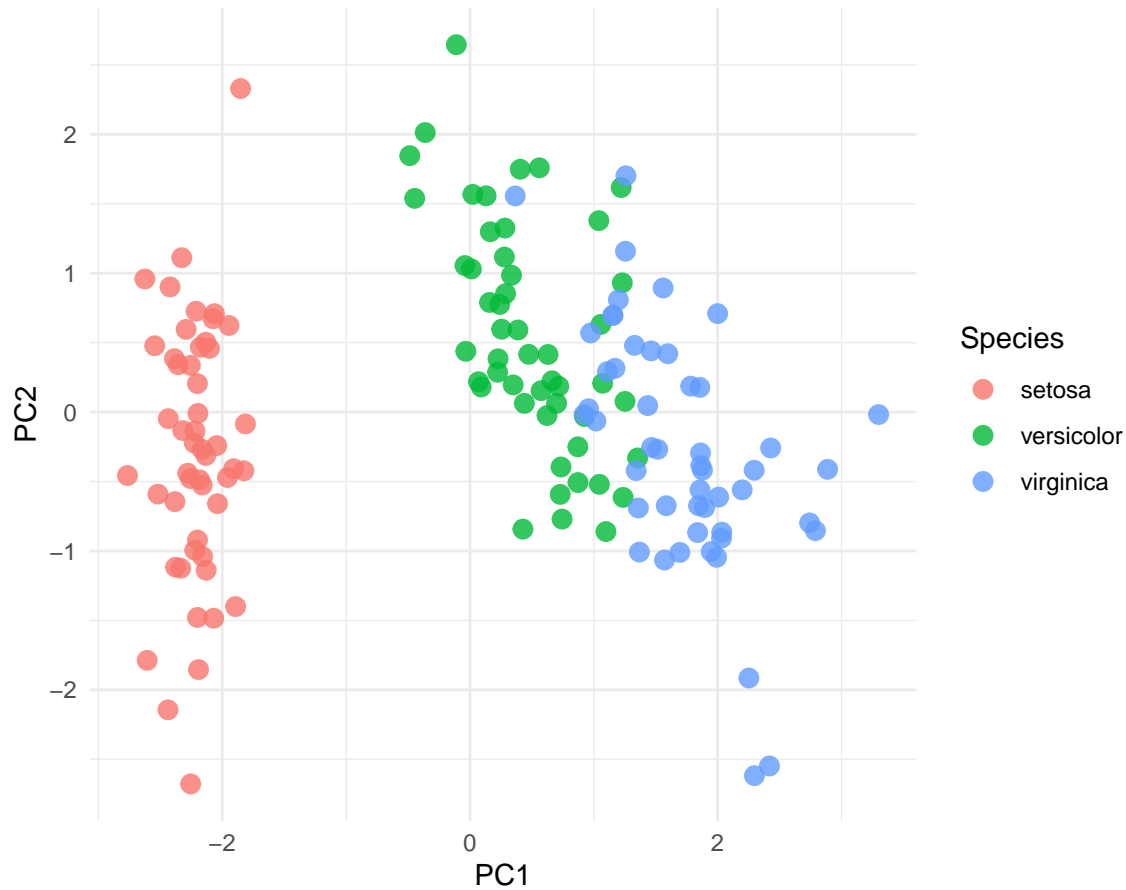
PCA of Iris dataset
