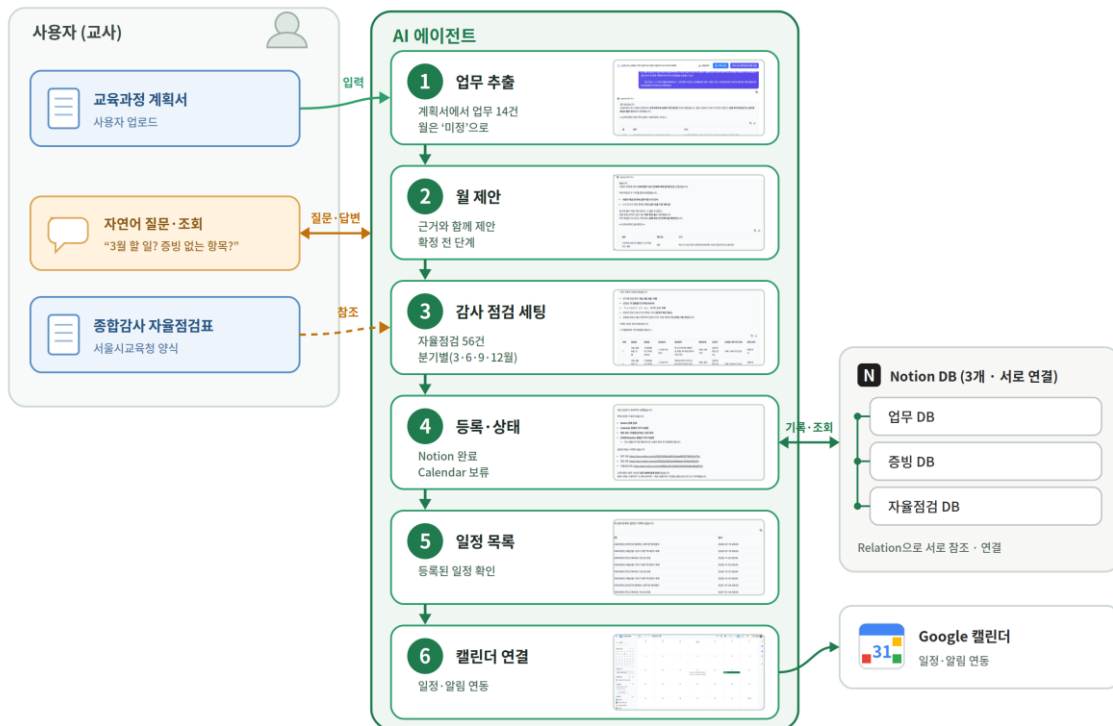
그림 5. 사용자와 AI 에이전트의 처리 흐름 (①~⑥은 아래 화면과 대응)
