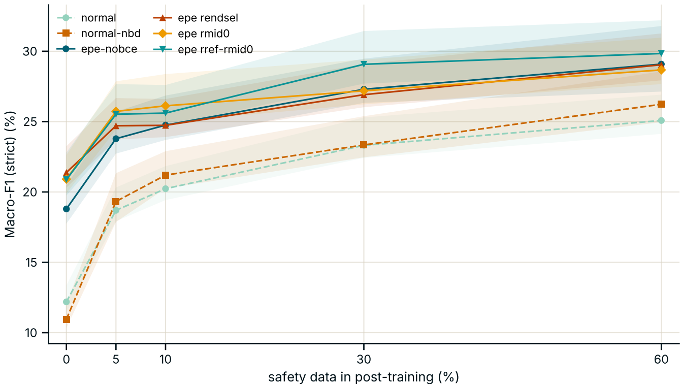
Macro-F1 (strict) vs safety-data mix
