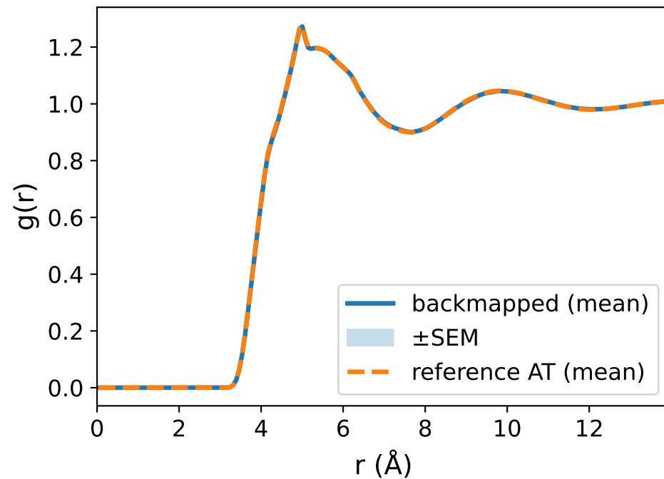
CH2-CH2
