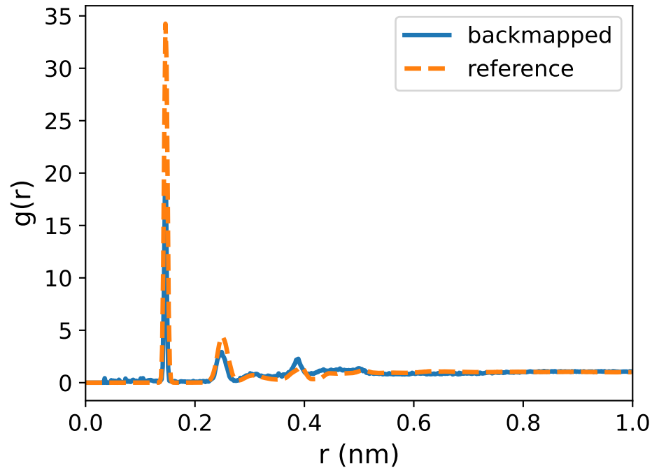
C-N vs AA
