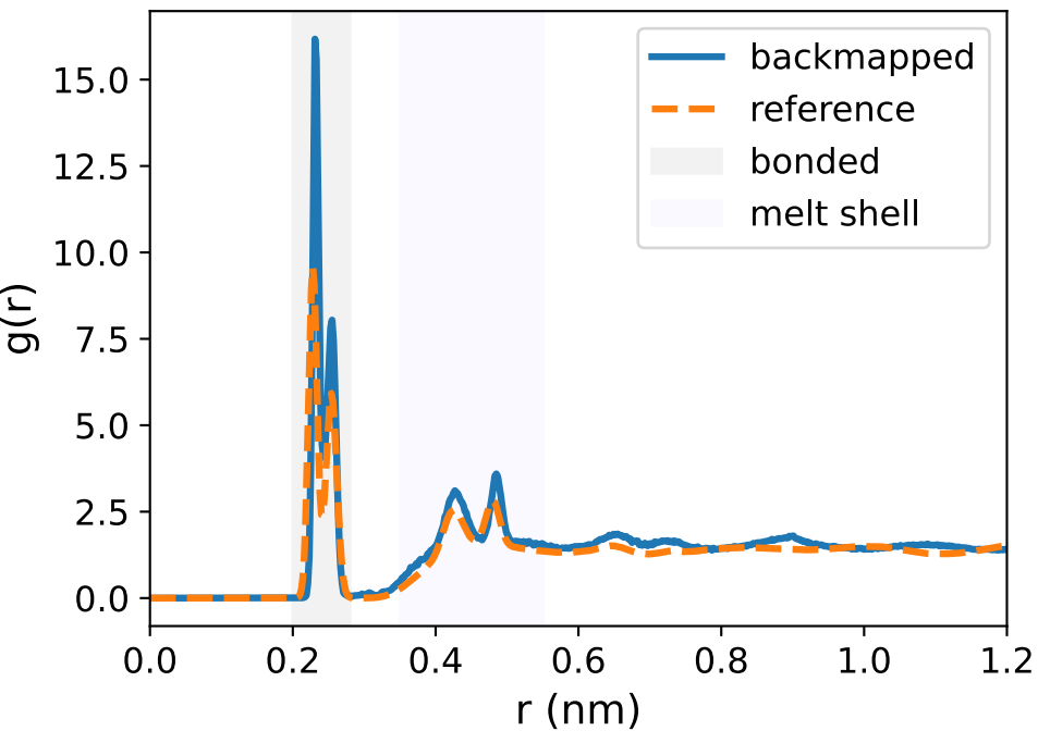
C-C
