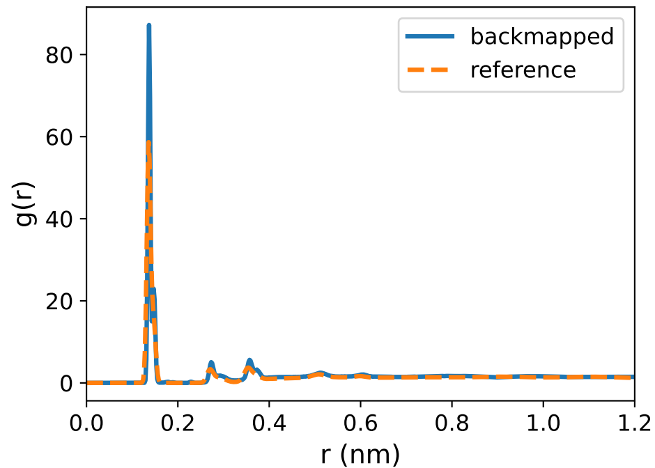
C-N
