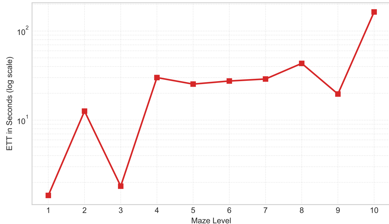
(B) Expected Time to Target (ETT)
