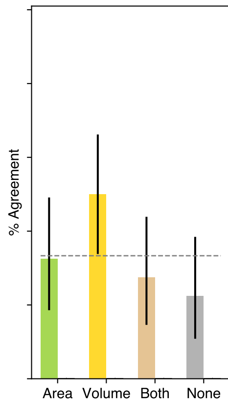
claude-2
