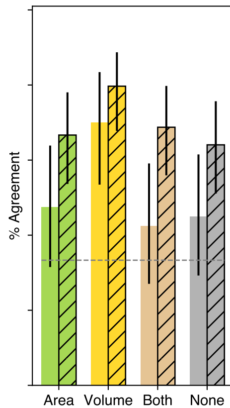
claude-3
