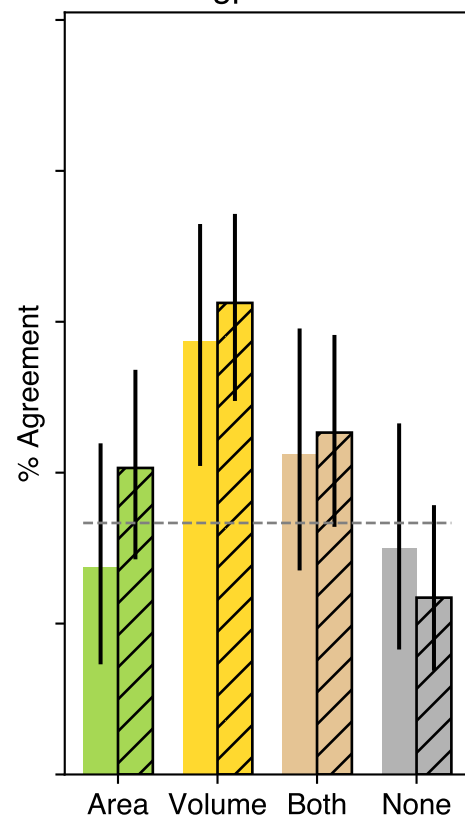
gpt-3.5
