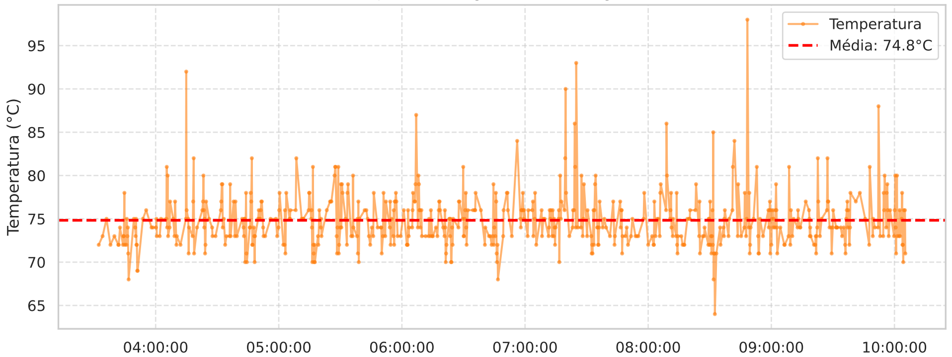
Evolução da Temperatura - Script: Threading
