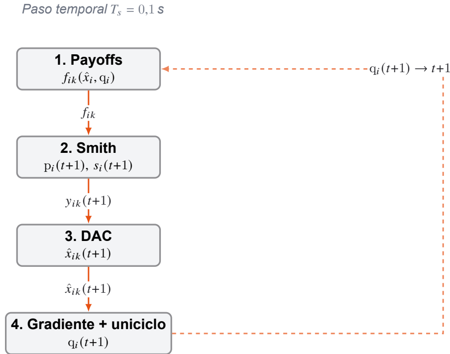
Figura 5. Bucle de control de las tres dinámicas acopladas. Los cuatro bloques se ejecutan secuencialmente dentro del mismo paso temporal T_s = 0,1 \text{ s} . La flecha discontinua representa la transición al instante siguiente t+1 .
