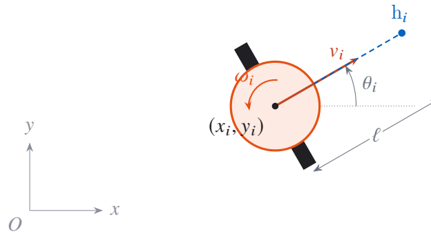
Figura 3. Modelo de robot móvil de tracción diferencial (unicycle). El estado es la pose q_i = (x_i, y_i, \theta_i) ; las entradas de control son la velocidad lineal v_i y la velocidad angular \omega_i . El punto adelantado h_i , situado a una distancia \ell del centro en la dirección de avance, es el que regula la ley de navegación reactiva (ec. 14).
