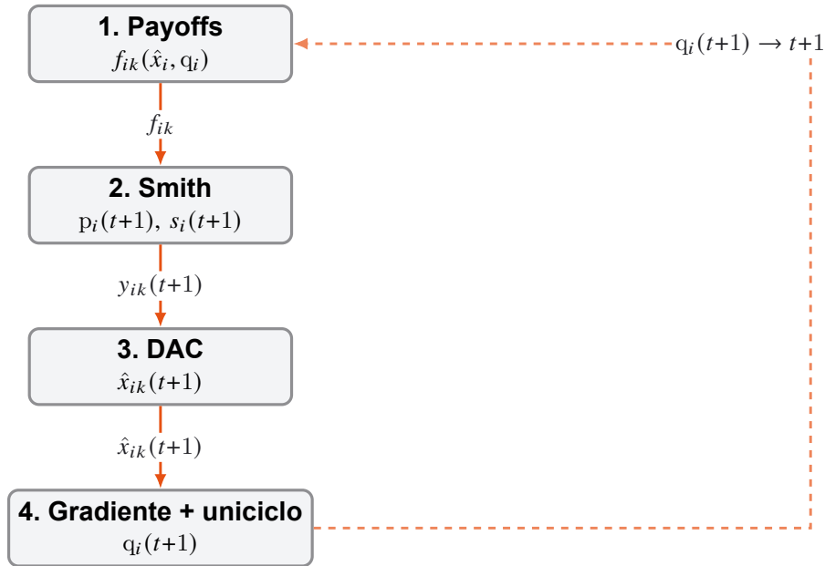
Figura 5. Bucle de control de las tres dinámicas acopladas. Los cuatro bloques se ejecutan secuencialmente dentro del mismo paso temporal T_s = 0,1 \text{ s} . La flecha discontinua representa la transición al instante siguiente t+1 .
