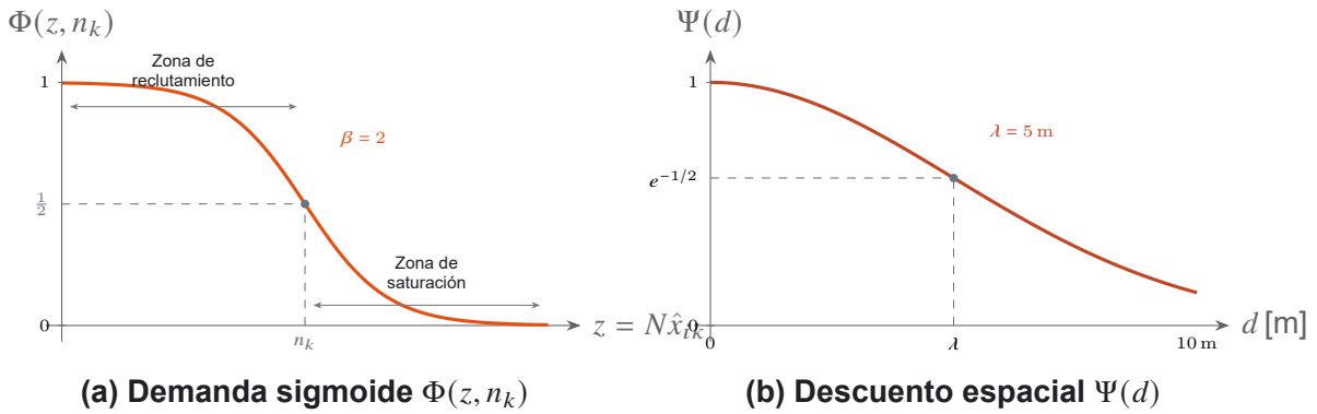
Figura 4. Componentes de la función de payoff (4). (a) La demanda sigmoide \Phi(z, n_k) es monótonamente decreciente: cuando el número estimado z = N \hat{x}_{ik} está por debajo de n_k , el payoff es alto (zona de reclutamiento); cuando supera n_k , cae a cero (zona de saturación). (b) El descuento gaussiano \Psi(d) reduce el payoff de robots lejanos de la tarea, integrando la dinámica espacial en el juego de asignación.
