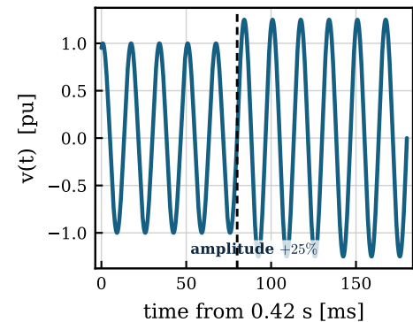
A Magnitude step
