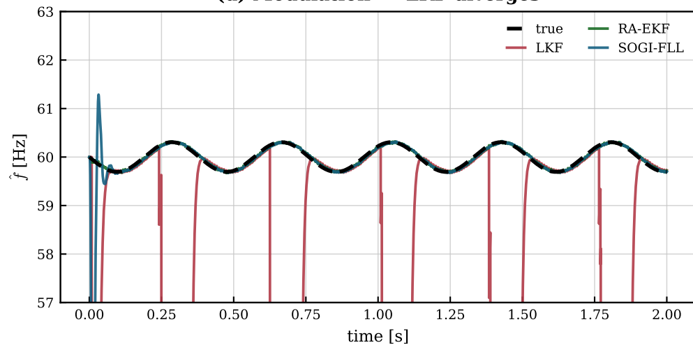
(d) Modulation --- LKF diverges
