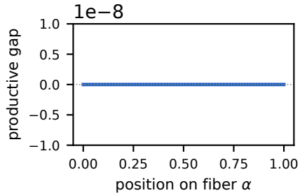
(a) V(z(\alpha)) - V^*
