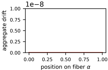
(b) \|Bz(\alpha) - y^*\|
