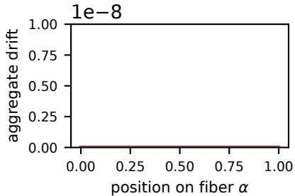
(b) \|Bz(\alpha) - y^*\|
