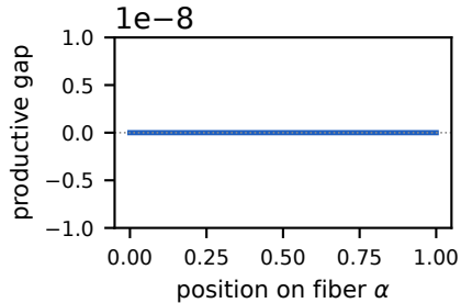
(a) V(z(\alpha)) - V^*
