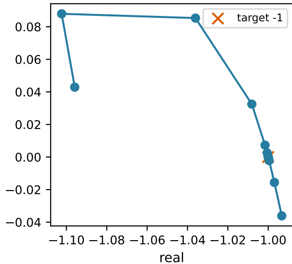
Q_H eigenvalue
