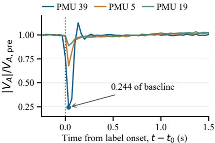
(d) Load change at bus 7
