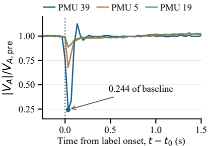
(d) Load change at bus 7
