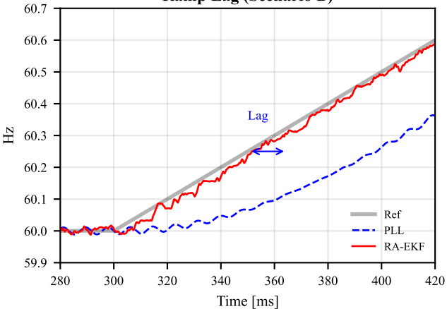
Ramp Lag (Scenario B)
