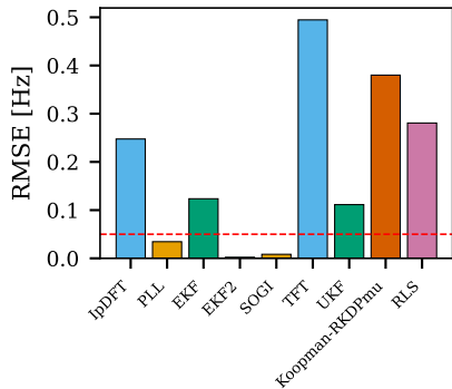
C1_VoltageSag
